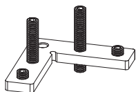
Längsverbinder 90° mit Arretierung und Kederklemmung Bestell-Nr.: V8R.LG-00ANK-90
