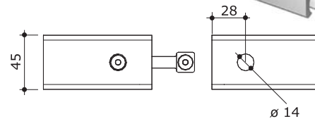
Längsverbinder - Hohlkammer
